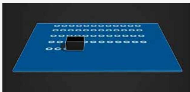
Рис. 2. Схема работы технологии MJM на прямоугольном / квадратном столе, компания dp Polar GmbH [2]
