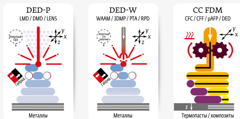
Рис. 5. Схемы использования в АП круглых вращающихся столов [1]
