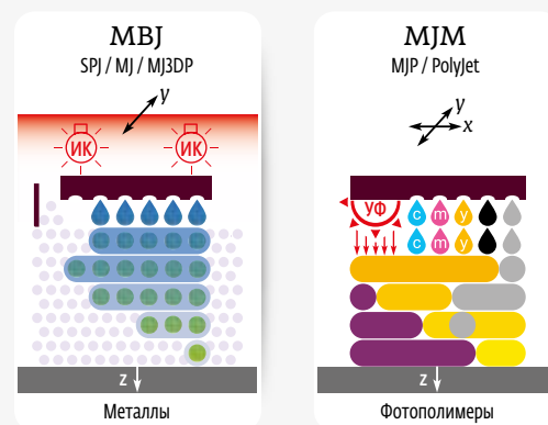
Рис. 8. Схема уникальной гибридной технологии на основе схем технологий MJM и MJB [1]
